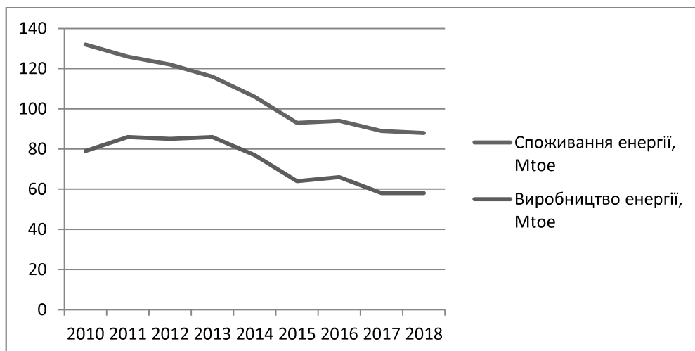
Рис. 2. Динаміка показників виробництва і споживання енергії в Україні за 2010-2018 рр.
